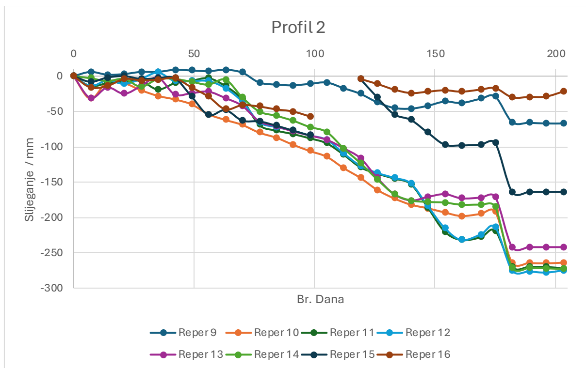
Slika 2. Prikaz slijezanja pojedinačnih repera (9-16) – Profil 2. (Nulto mjerenja: 11.7.2024.)
