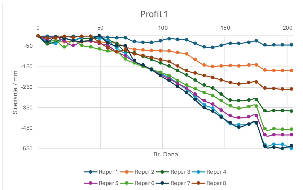
Slika 1. Prikaz slijezanja pojedinačnih repera (1-8) – Profil 1. (Nulto mjerenja: 11.7.2024.)
