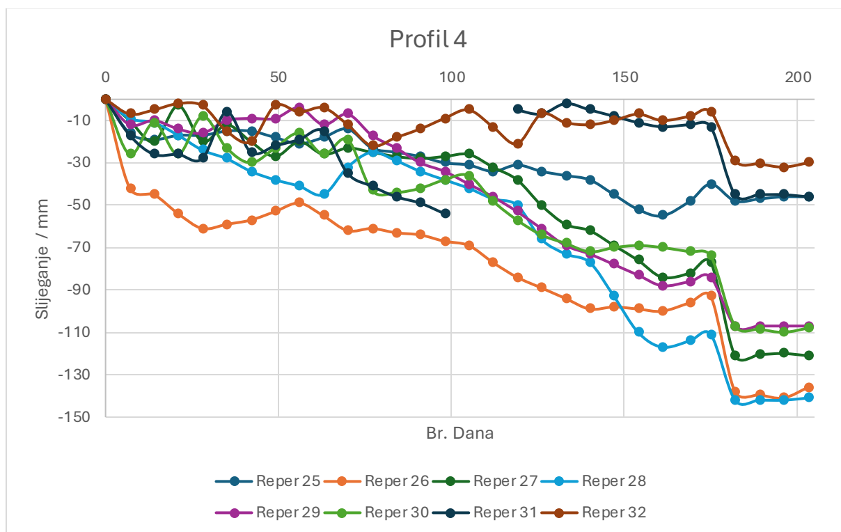
Slika 4. Prikaz slijeganja pojedinačnih repera (25-32) – Profil 4. (Nulto mjerenja: 11.7.2024.)
