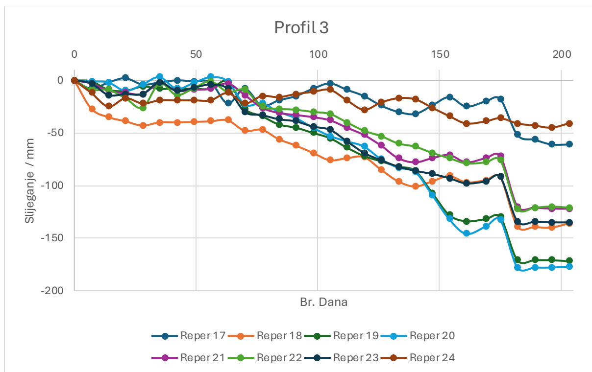
Slika 3. Prikaz slijeganja pojedinačnih repera (17-24) – Profil 3. (Nulto mjerenja: 11.7.2024.)
